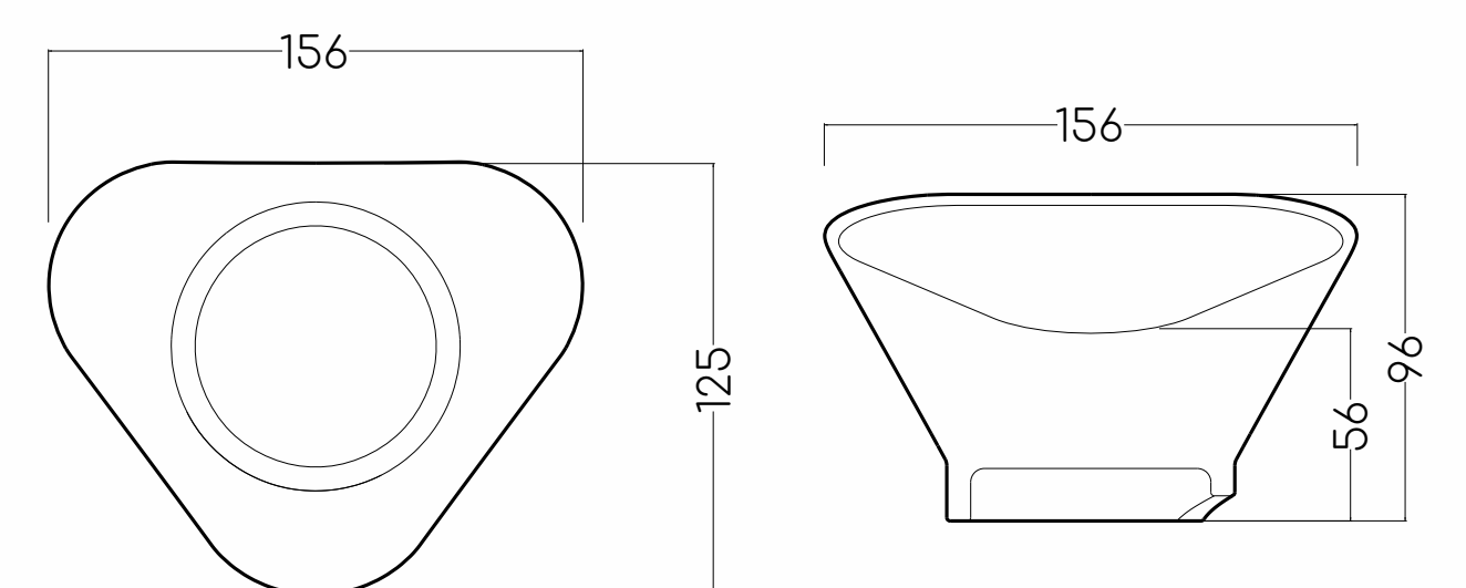
Rozměry misky na vodu
